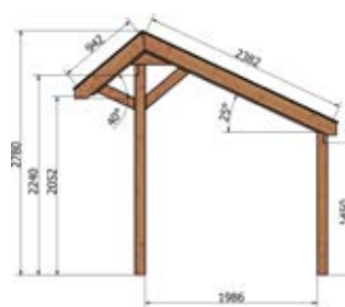
Zijaanzicht L
