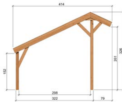
Zijaanzicht
